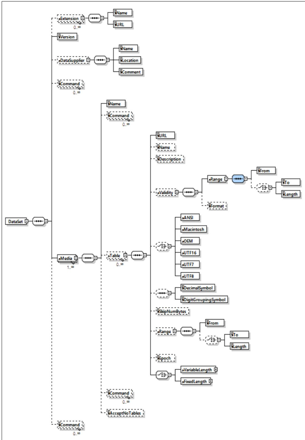
Abbildung 7: Beschreibungsstandard – DataSet
