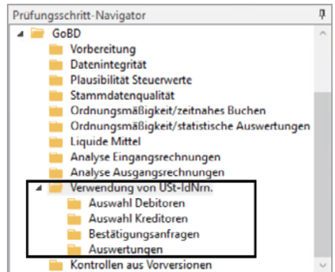
Neue Struktur der Kontrollen im Prüfungsschritt-Navigator
